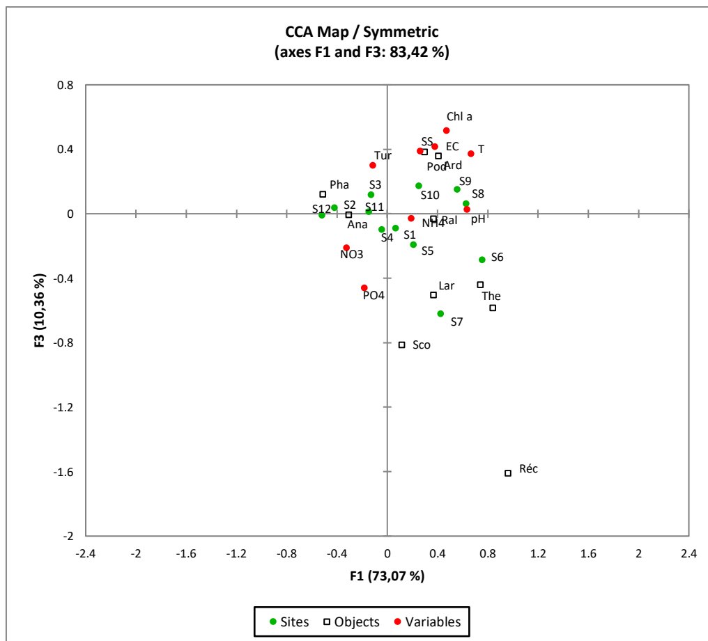
Figure 61. Représente les variables sur le plan factoriel 1x3 de la CCA (Analyse Canonical des Correspondances).
